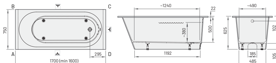
VARIO L 1700×750 mm 1600-1700×750 mm h = 625 mm Talpa: 220 l Svoris: 107 kg
