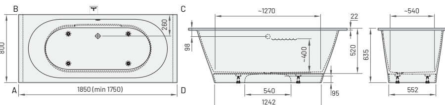
VARIO XL 1850×800 mm 1750-1850×800 mm h = 635 mm Talpa: 240 l Svoris: 135 kg
