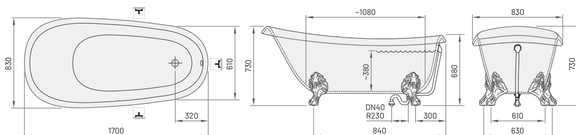
ANTICA (GRAPHITE) kojos
