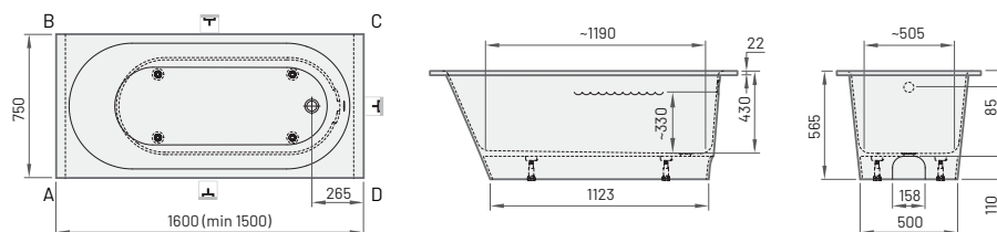
VARIO M 1600×750 mm 1500-1600×750 mm h = 565 mm Talpa: 200 l Svoris: 100 kg
